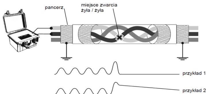
Rys. 36. Schemat podłączenia nadajnika i wykrycia miejsca zwarcia między żyłami
